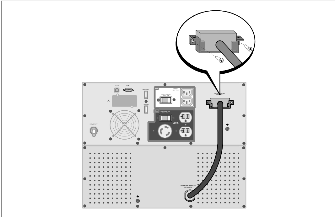
图 17. EBM 安装
