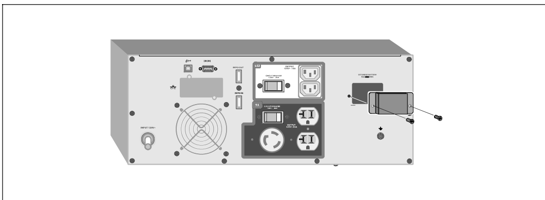
图 15. 取下电池连接器盖
