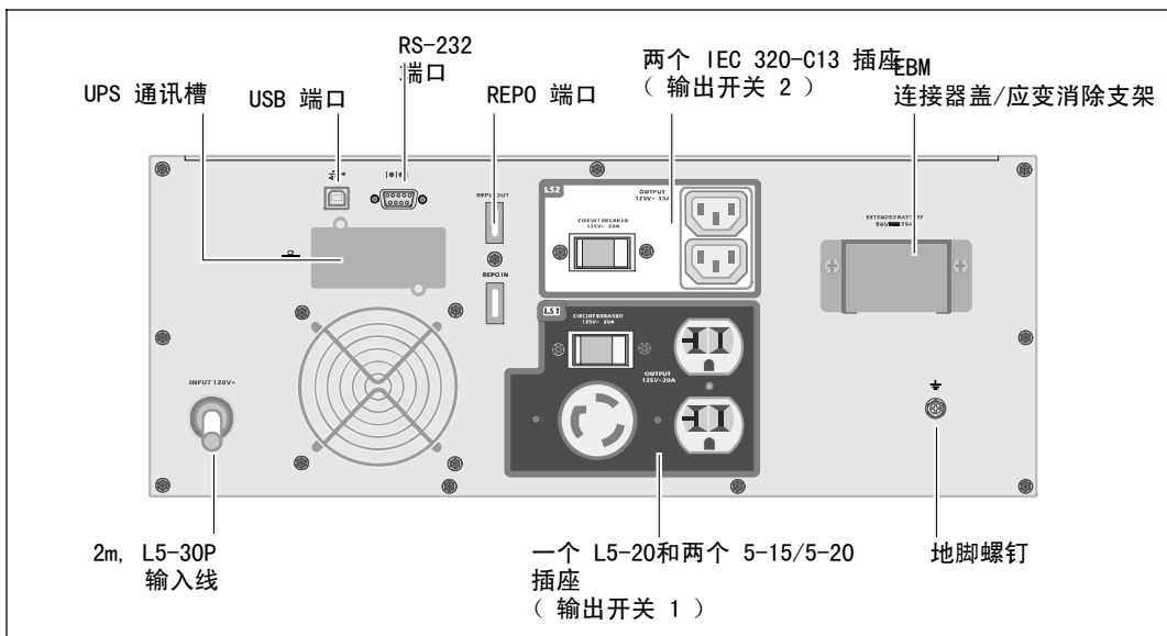
图 4. 2700W, 120V 后面板
