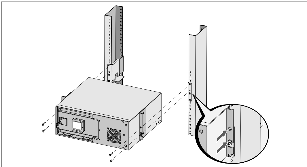
图 12. 安装和固定机箱
