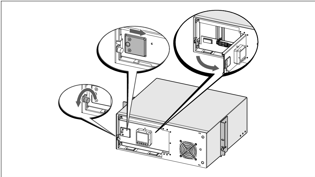
图 24. 打开电池金属盖
