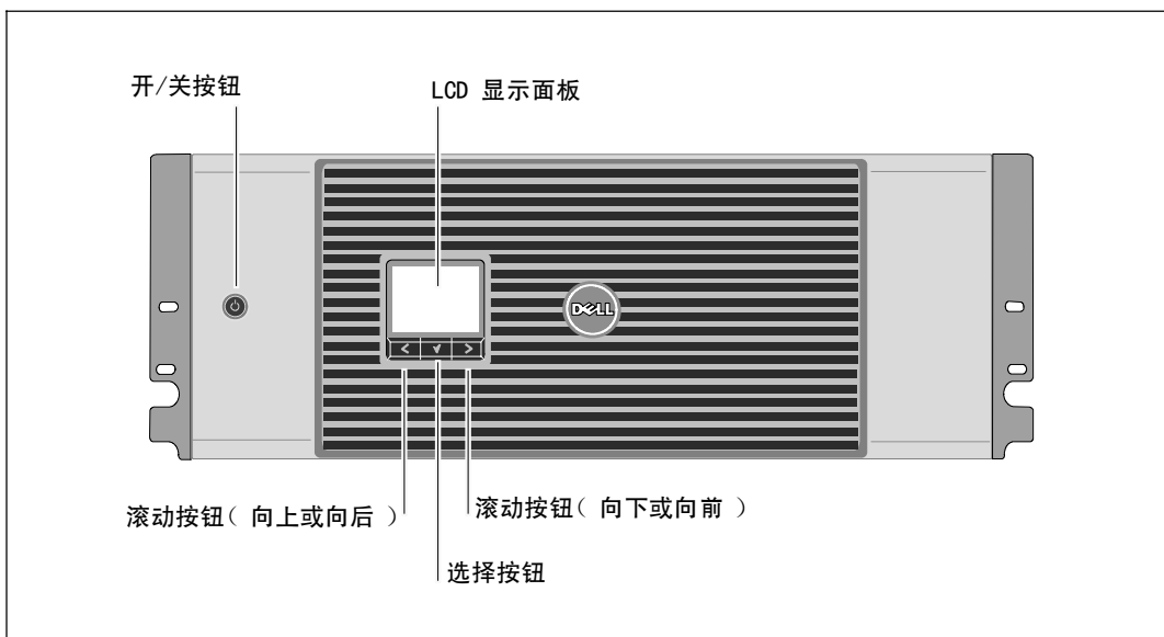
图 7. Dell 在线机架式 UPS 前面板
