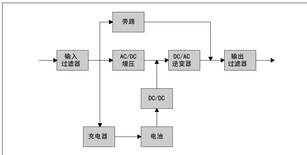
图 27. 在线 UPS 方框图
