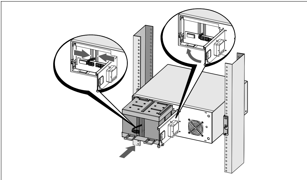
图 13. 安装电池座
