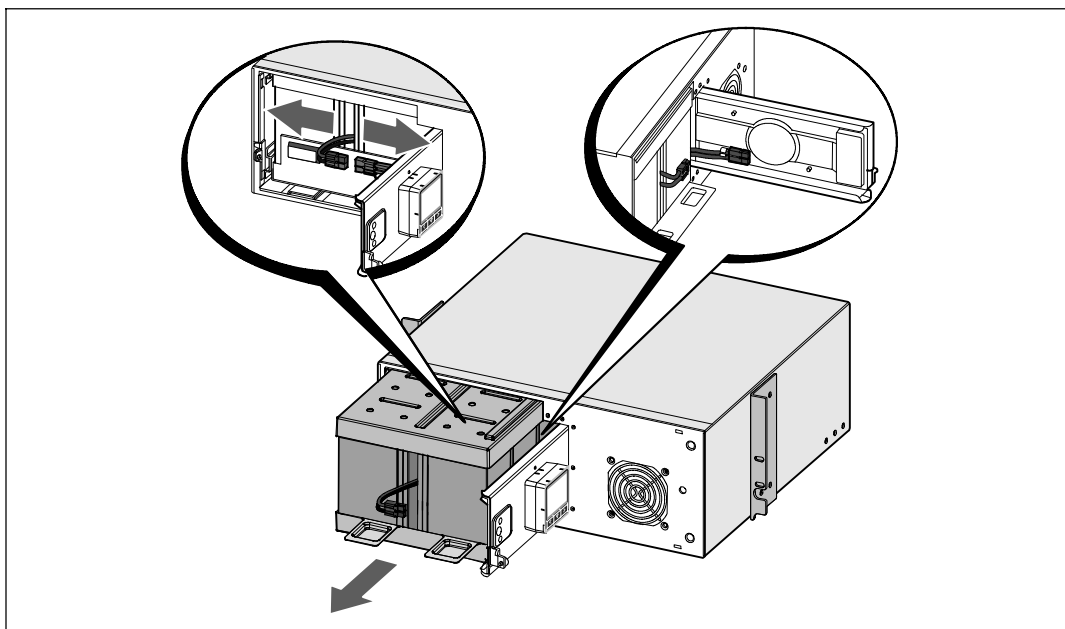
图 9. 取下电池座
