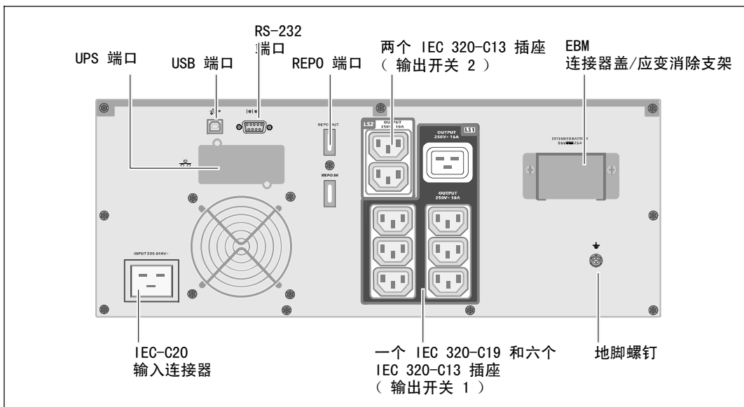
图 6. 2700W, 230V 后面板
