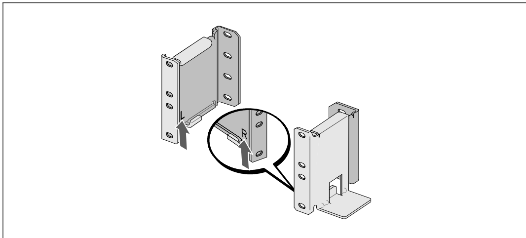
图 10. 定位导轨
