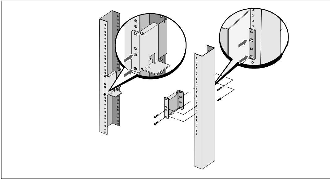
图 11. 将导轨连接到机架上
