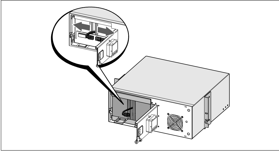
图 25. 断开 UPS 内置电池连接器
