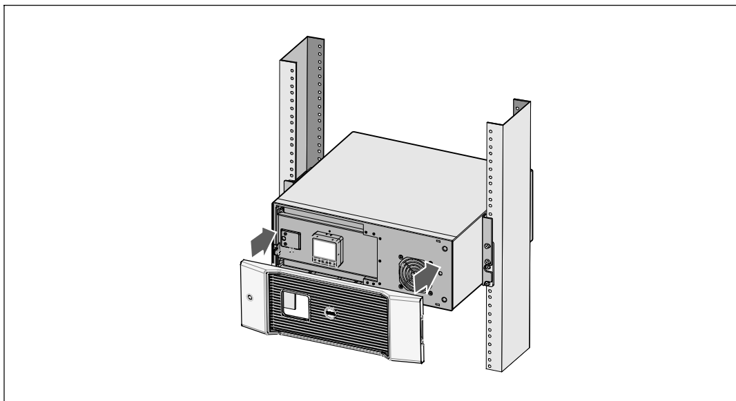
图 14. 安装 UPS 前盖
