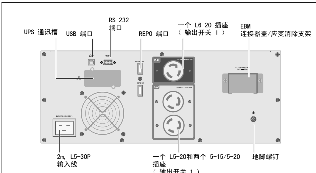
图 5. 2700W, 208V 后面板
